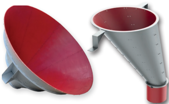
Trichterauskleidung aus einzelnen Segmenten mit Aluminium Lochblecheinlage
