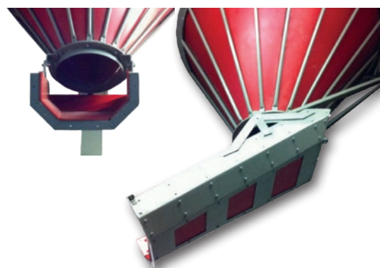
Stabtrichterauskleidung aus PUCEST Platten mit Verladerutsche und Inlay
